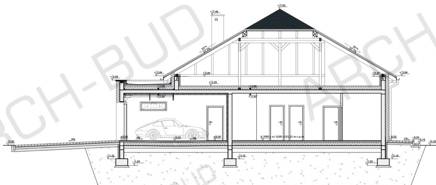
PRZEKRÓJ A-A
